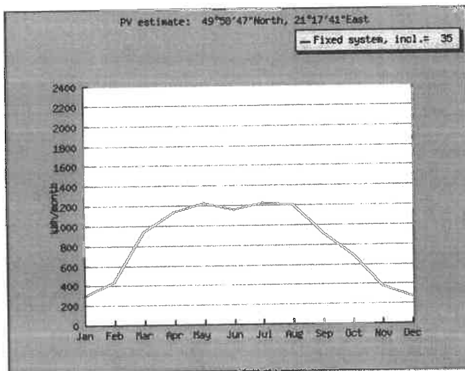
Wykres 4. Produkcja energii z systemu PV 10kWp.
